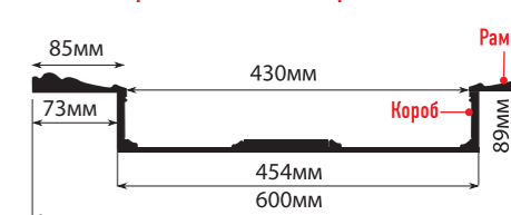
KS61A-19D рама: 600x600x25, короб: 454x454x89
